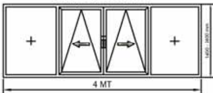
480497 (380497) ŞEMA C / 2 MT RAY
