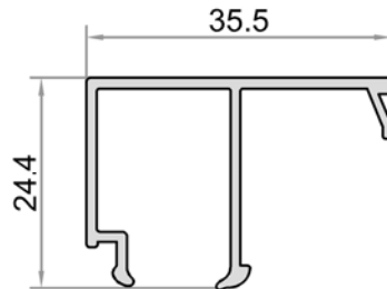
W-516-a AĞIRLIK / WEIGHT (KG/M.) 0,265
